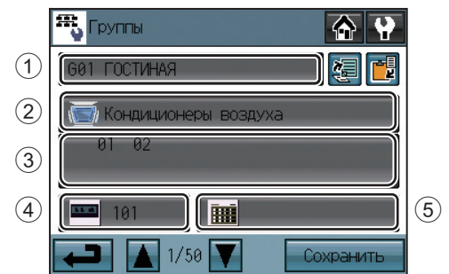
Экран настройку группы
