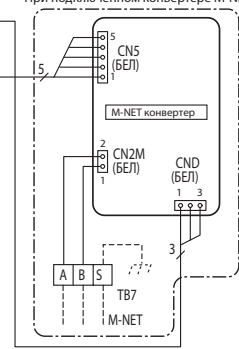
При подключенном конвертере M-NET
