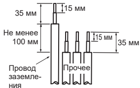
Шнур источника питания (К)
